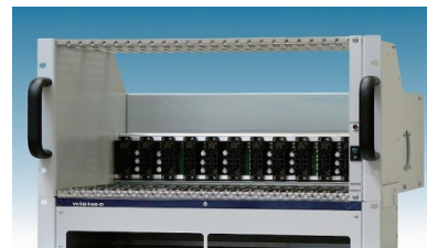
ファンあり7Uタイプ
