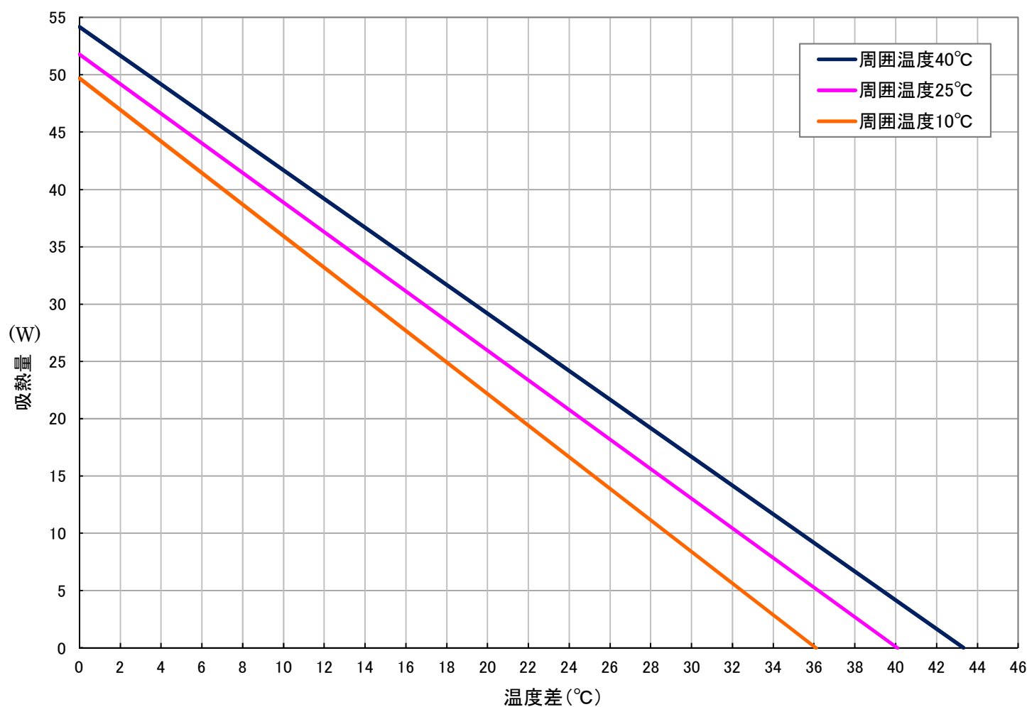
HMC-19F-0400 / HMC-19F-0420 温度差と吸熱量
