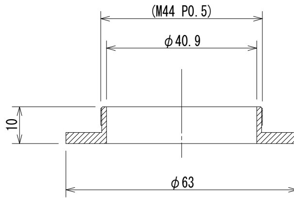
A-A断面
