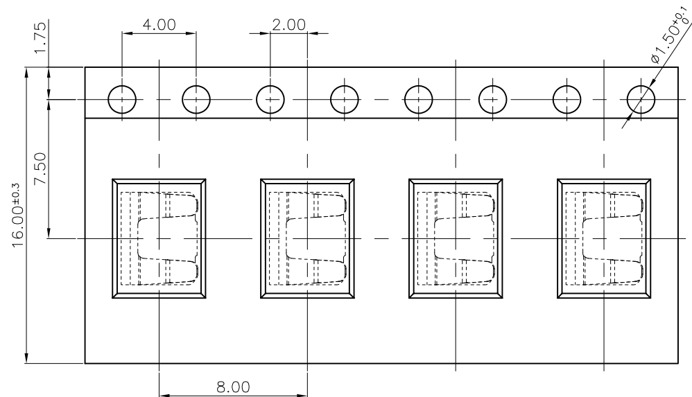
Reel Tray S=5:1
